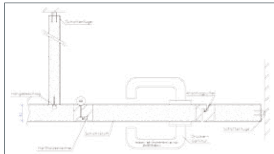
DETAIL: Horizontalschnitt HS V
