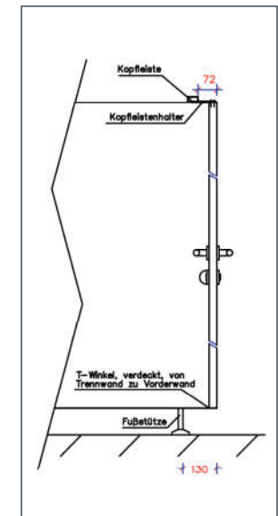
DETAIL: Vertikalschnitt S30 Fly
