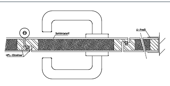
DETAIL: Türquerschnitt S30
