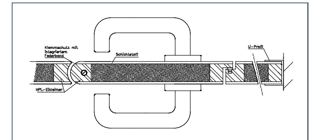
DETAIL: Türquerschnitt S30/ KL mit Schattenfuge
