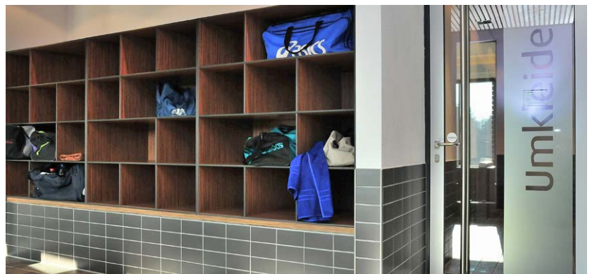
/// Oben: Individuell gefertigte Ablagefächer und Wandverkleidungen aus HPL, Dekor Zebrano, im Saunabereich. Unten links: Ablage mit Hakenleiste aus Aluminium im Duschbereich der Saunen. Unten rechts: Zwischen den Umkleideräumen und den Saunabereichen bieten großzügige Ablagefächer ausreichend Platz für Handtücher, Taschen etc.
