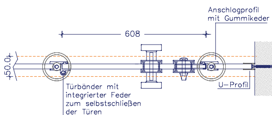
Horizontalschnitt
