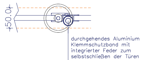
bandseitiger Klemmschutz
