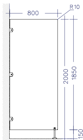
Sichtschutzwand
