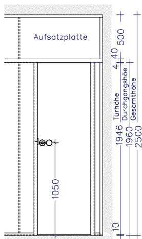
raumhohe Ausführung
