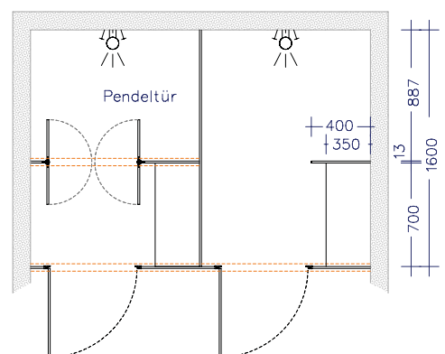
Duschkabine
